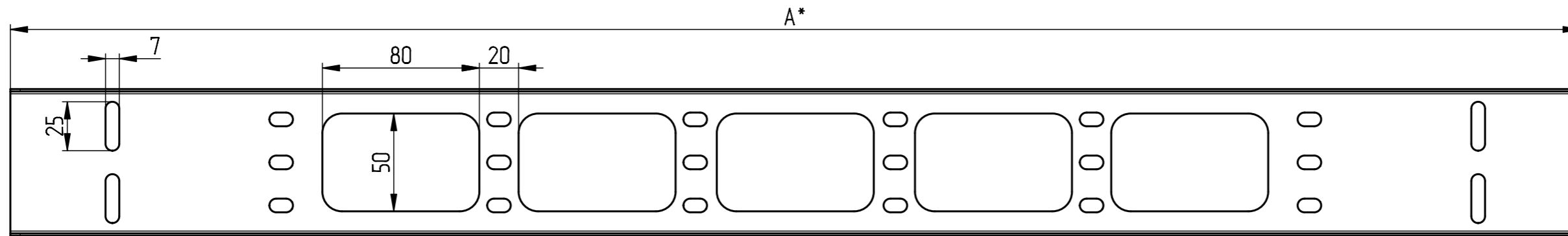
Рис.2 остальное см. рис.1 M1:4
